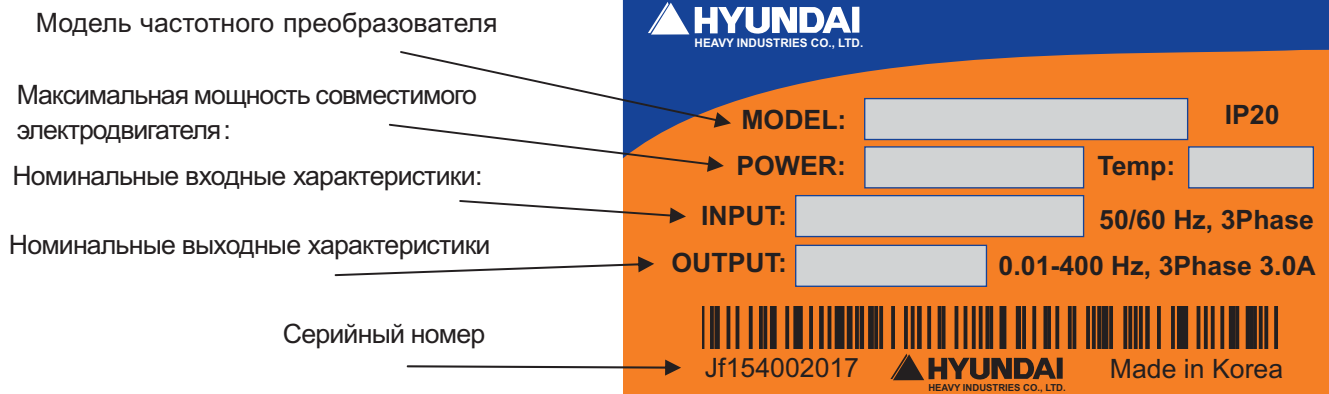
Рисунок 1-2: Содержание заводской таблички
