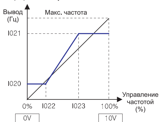
Рис. 9-26 Установка пусковой частоты в установке клеммы O-L
