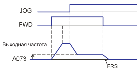
Рис. 7-7 Кривая выбора толчкового функционирования
