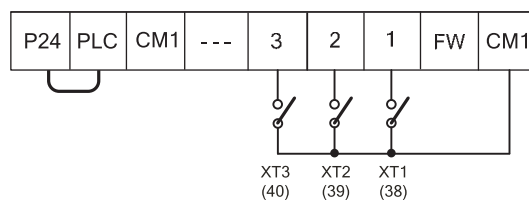
Рис. 9-25 Выбор функции установки времени многоскоростного ускорения/замедления
