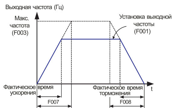
Рис. 6-1 Кривая установки выходной частоты
