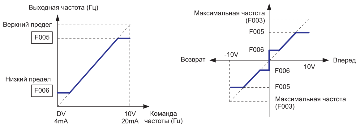
Рис.6-5 Пределная кривая частоты (при использовании O-L,OI-L)
