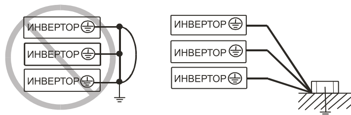
Рис. 2- 6 Заземление (G)
