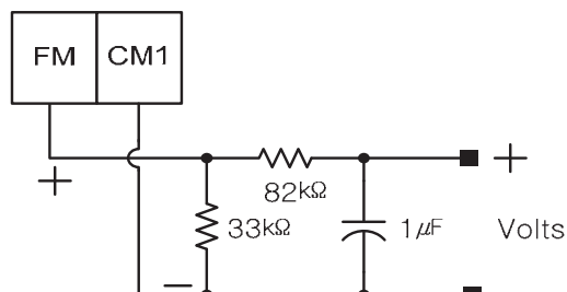
Рис. 10-15 Когда выходная частота – 60Гц, откалибруйте величину о011 чтобы измеритель показывал 60Гц.
