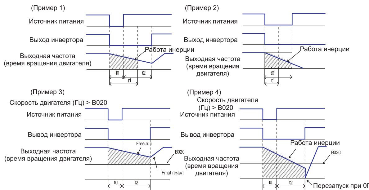
Рис. 8-2 Пример пуска при соответствии частоты
