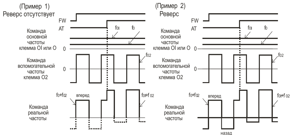
Рис. 9-20 Пример выбора аналогового внешнего сигнала
