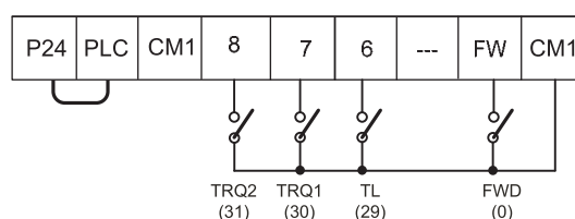
Рис. 11-3 Установка предела вращающего момента в микропроцессорной входной клемме
