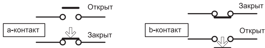
Рис. 10-3 Схема функционирования контакта а и контакта b
