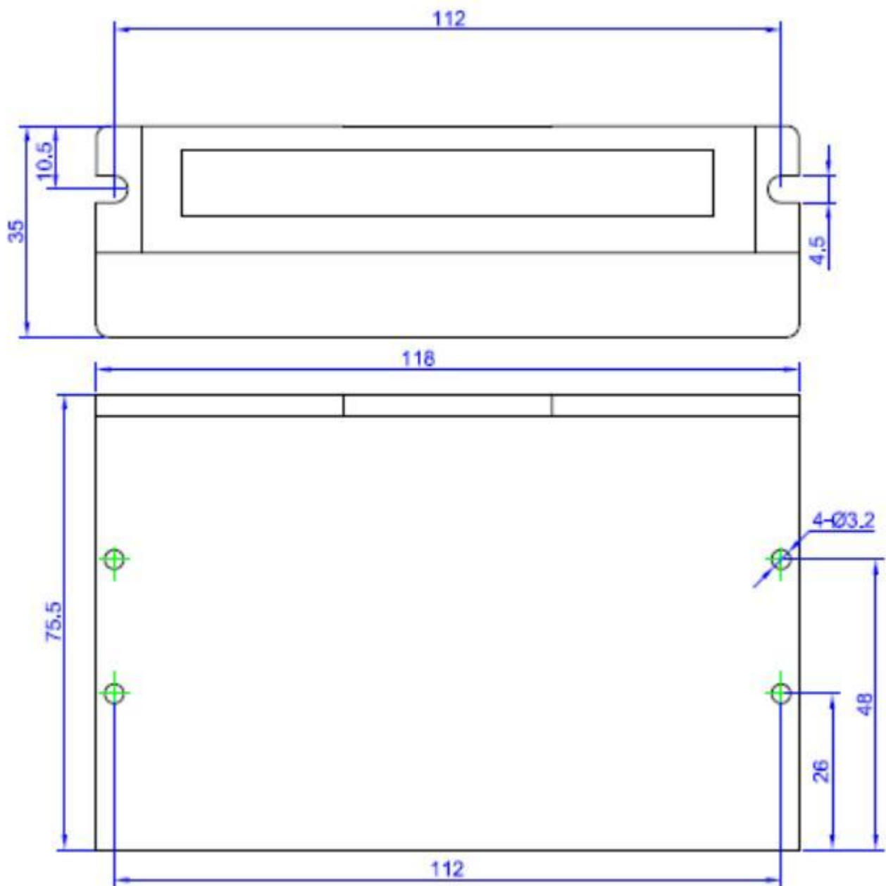
Рис.3. Монтажные размеры
