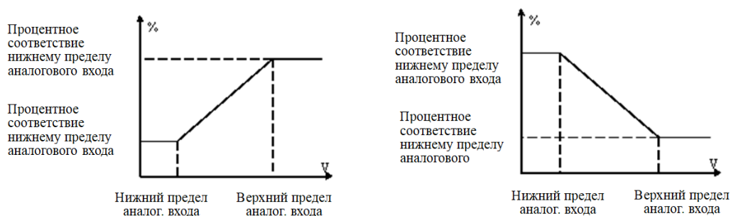
Рис. 6-18 Линейная кривая аналогового входа
